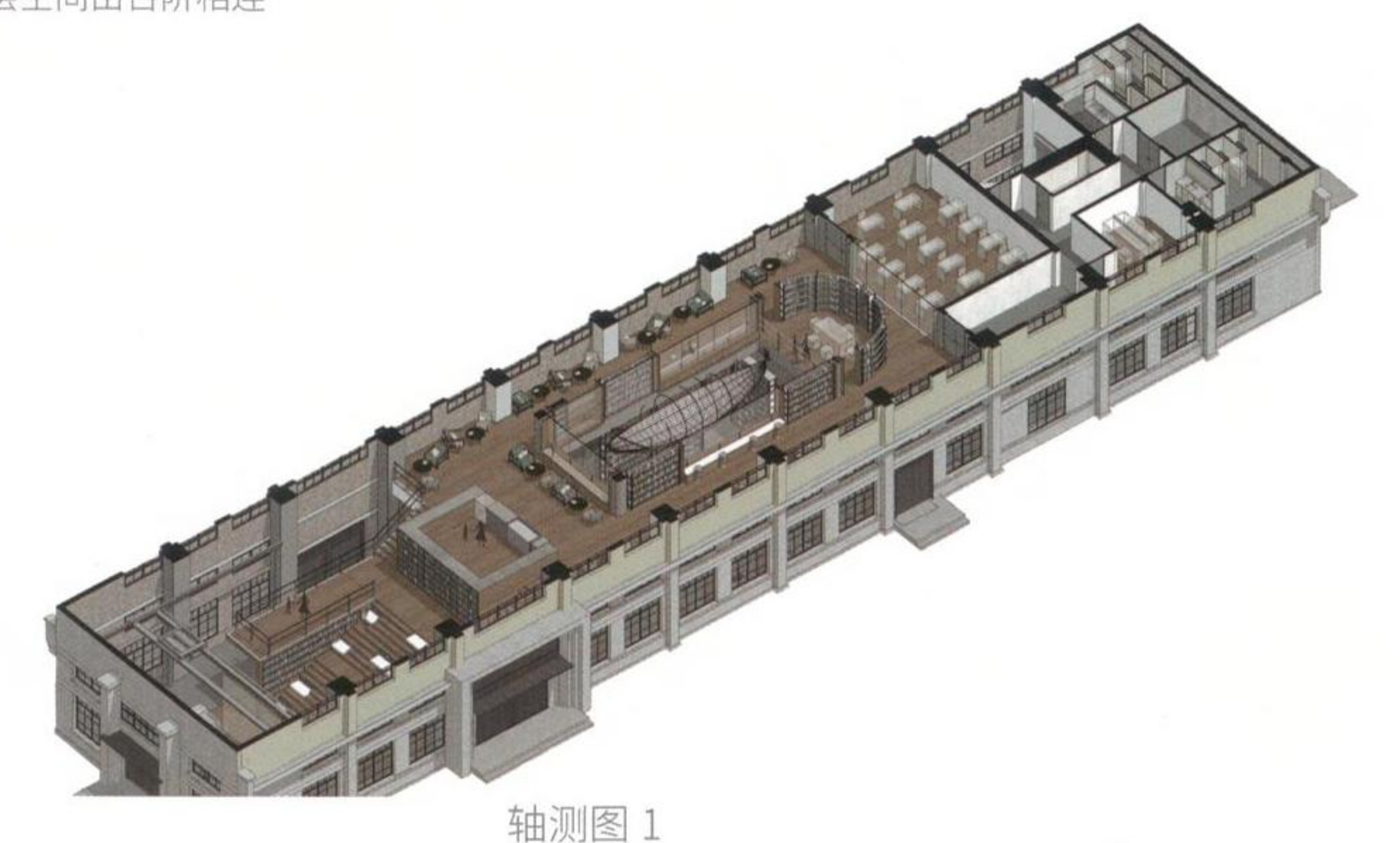
轴测图 1
